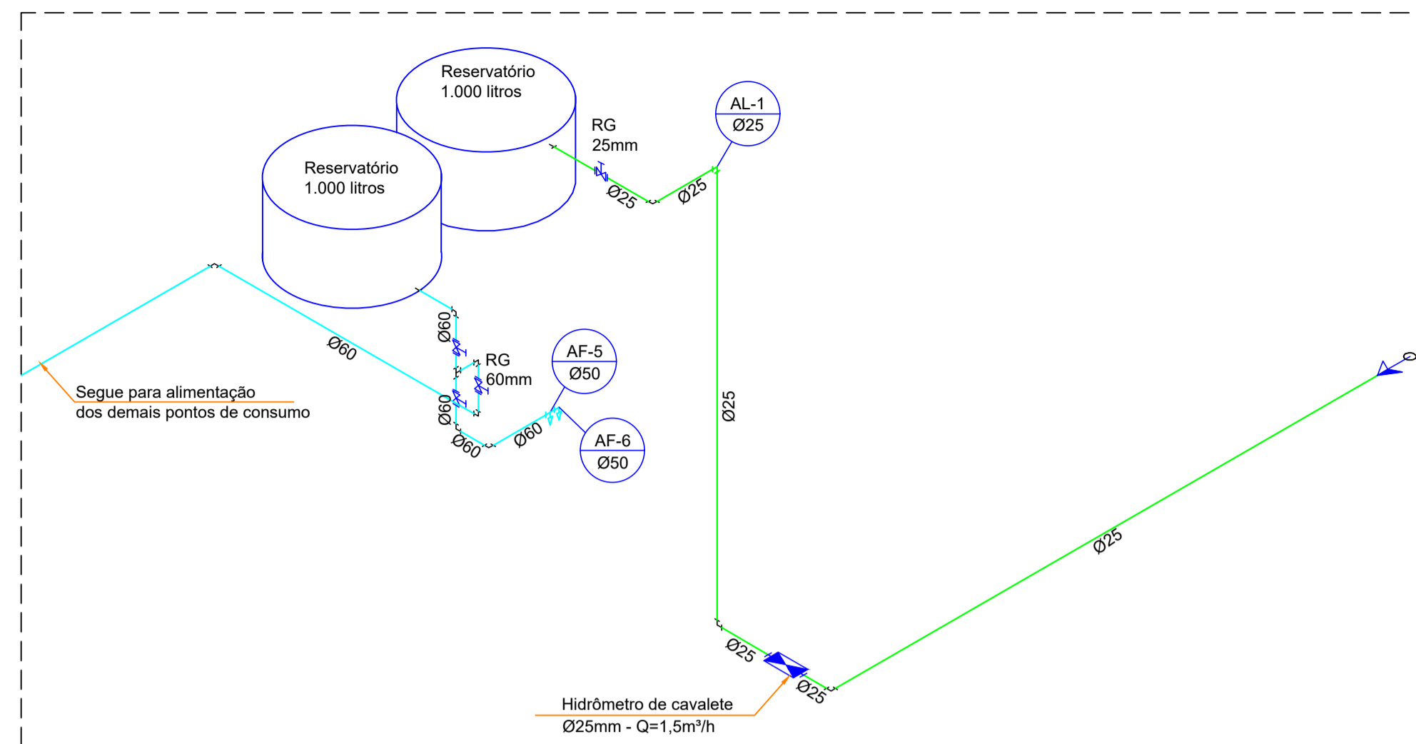
Isométrico - Reservatório Escala: 1/50
