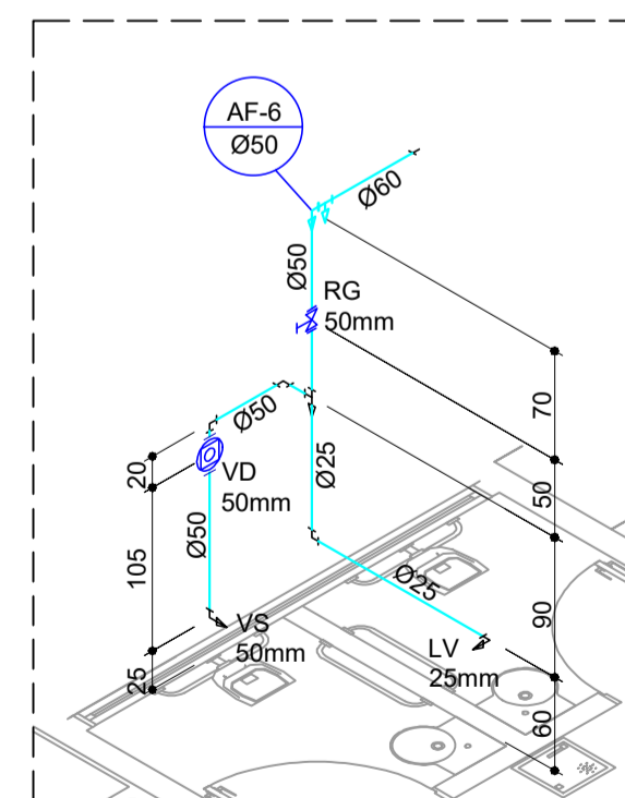
Detalhe - D05 Escala: 1/50
