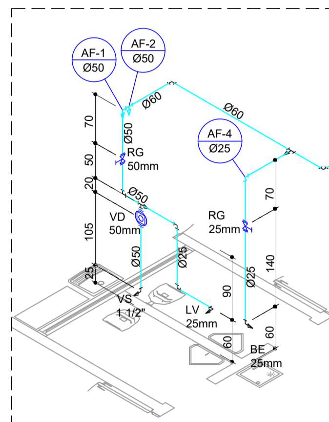
Detalhe - D02 Escala: 1/50
