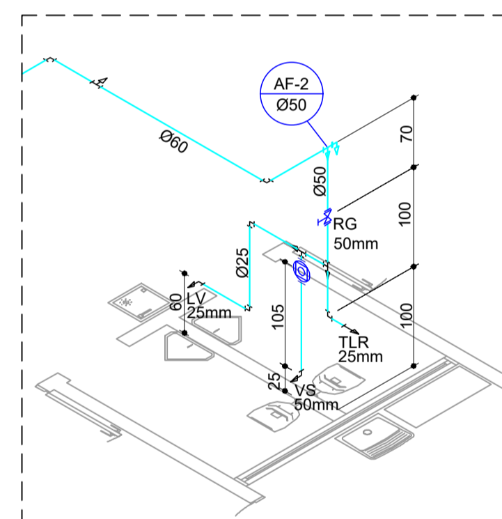
Detalhe - D01 Escala: 1/50
