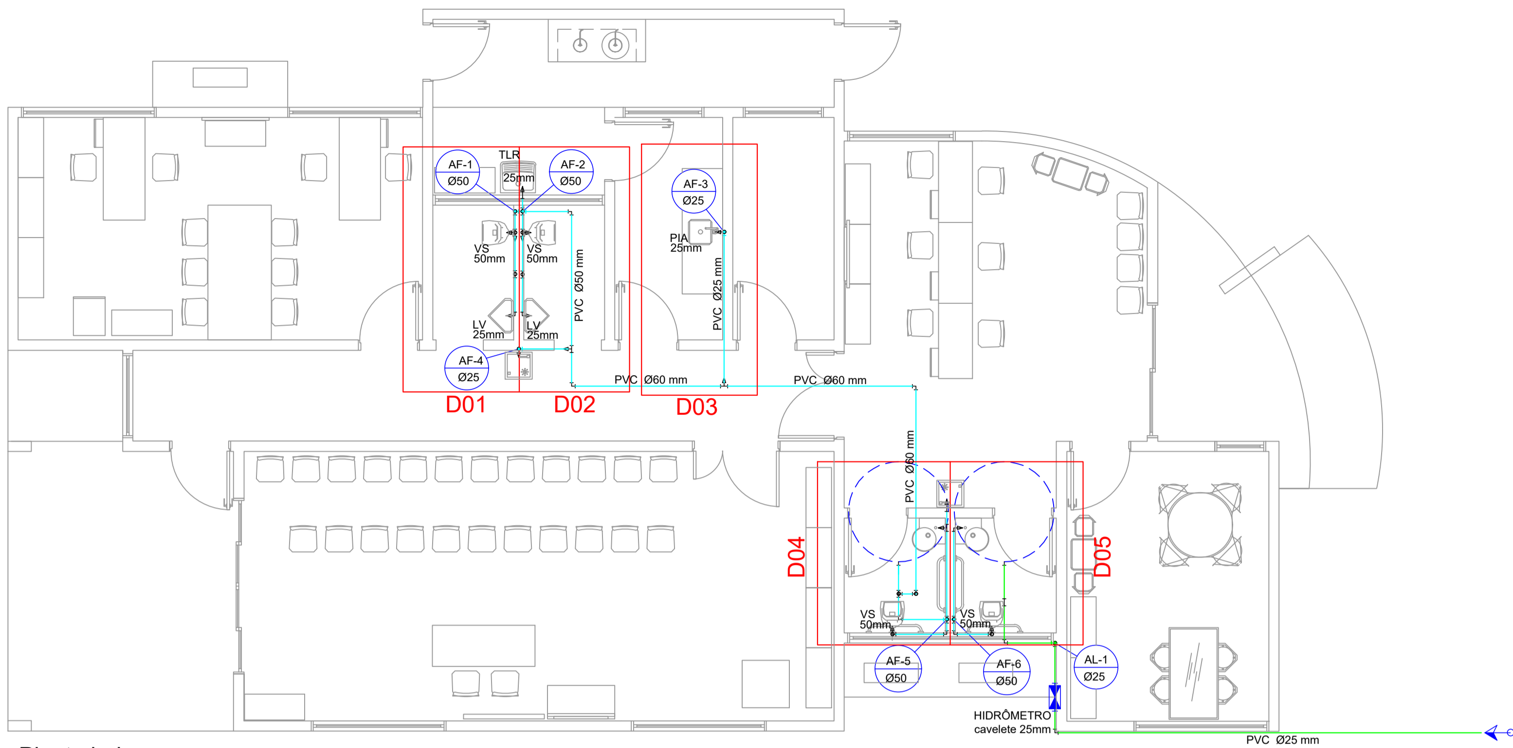
Planta baixa Área: 165,30 m 2 Escala: 1/50
