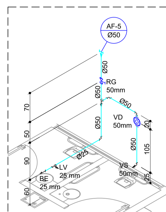
Detalhe - D04 Escala: 1/50
