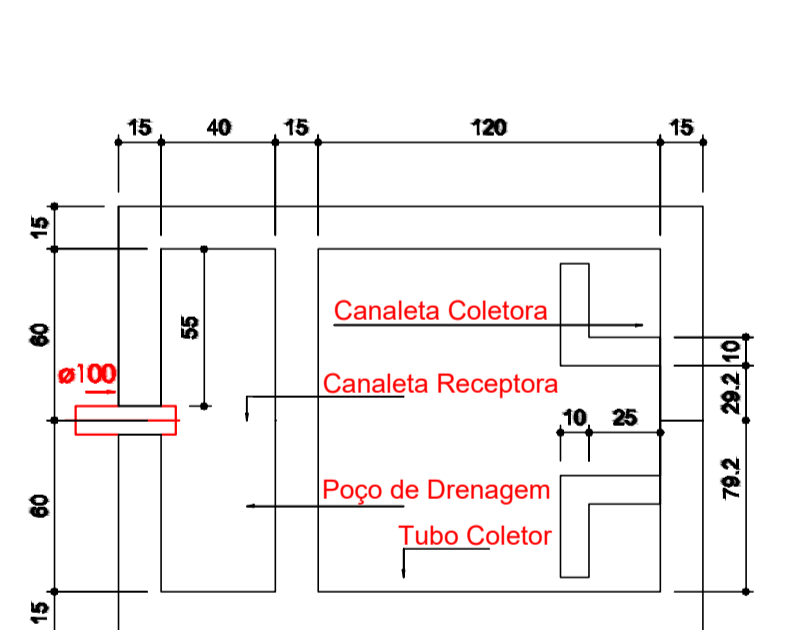
Filtro Anaeróbico - Planta Baixa Escala: 1/25
