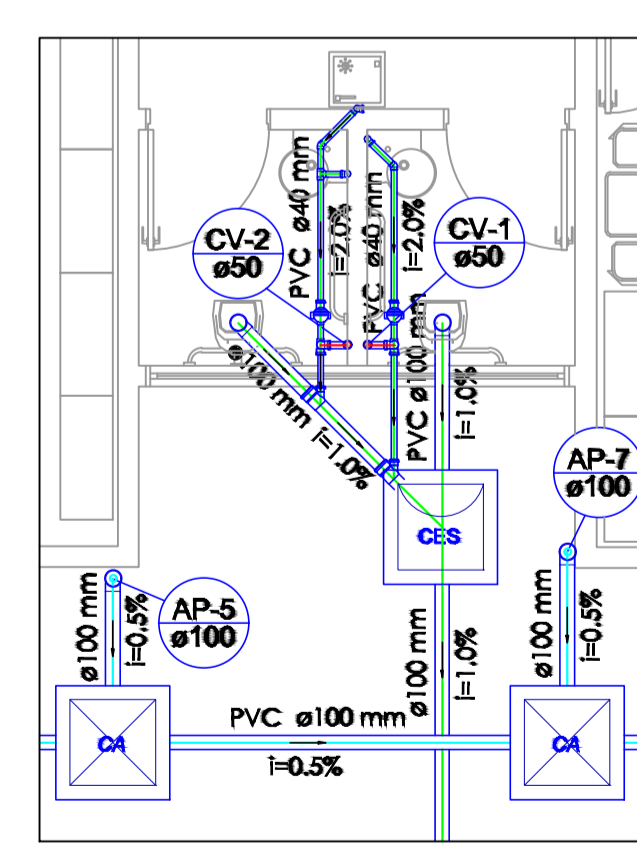
Detalhe - S2 Escala: 1/50
