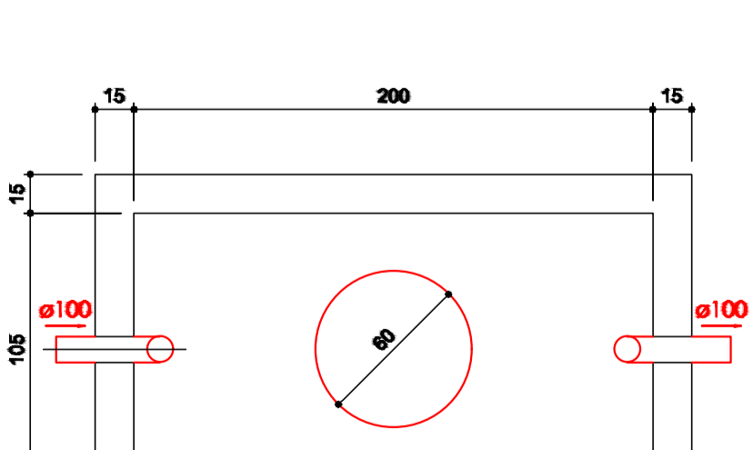
Tanque séptico - Planta baixa Escala: 1/25
