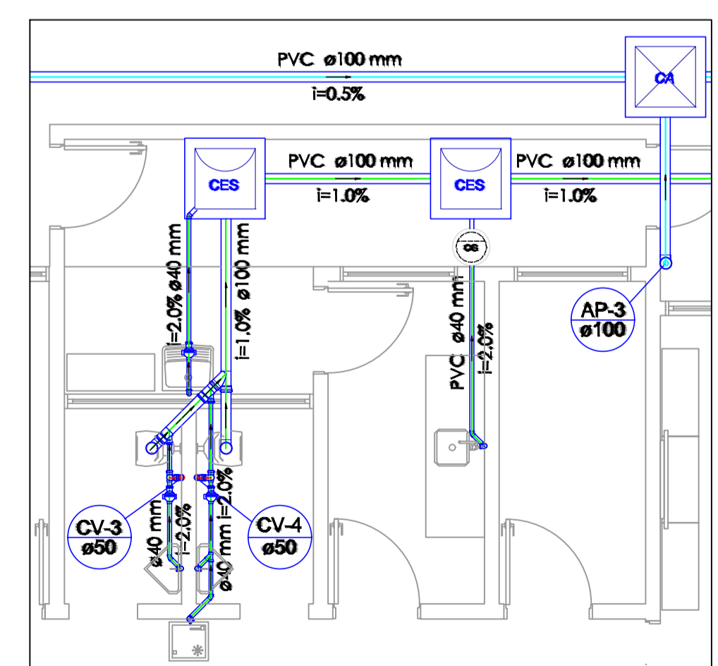
Detalhe - S1 Escala: 1/50
