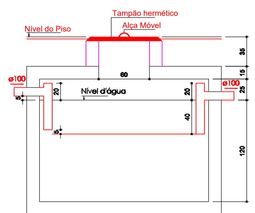
Tanque séptico - Corte Escala: 1/25
