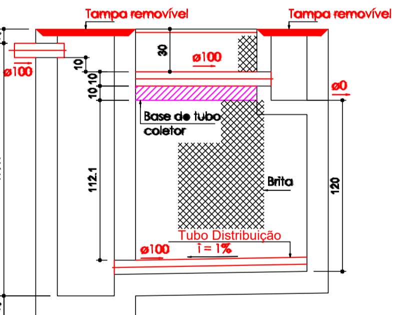
Filtro Anaeróbico - Corte Escala: 1/25
