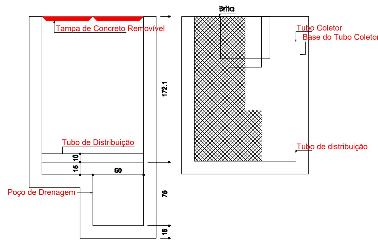
Tanque Anaeróbico - Corte Escala: 1/25
