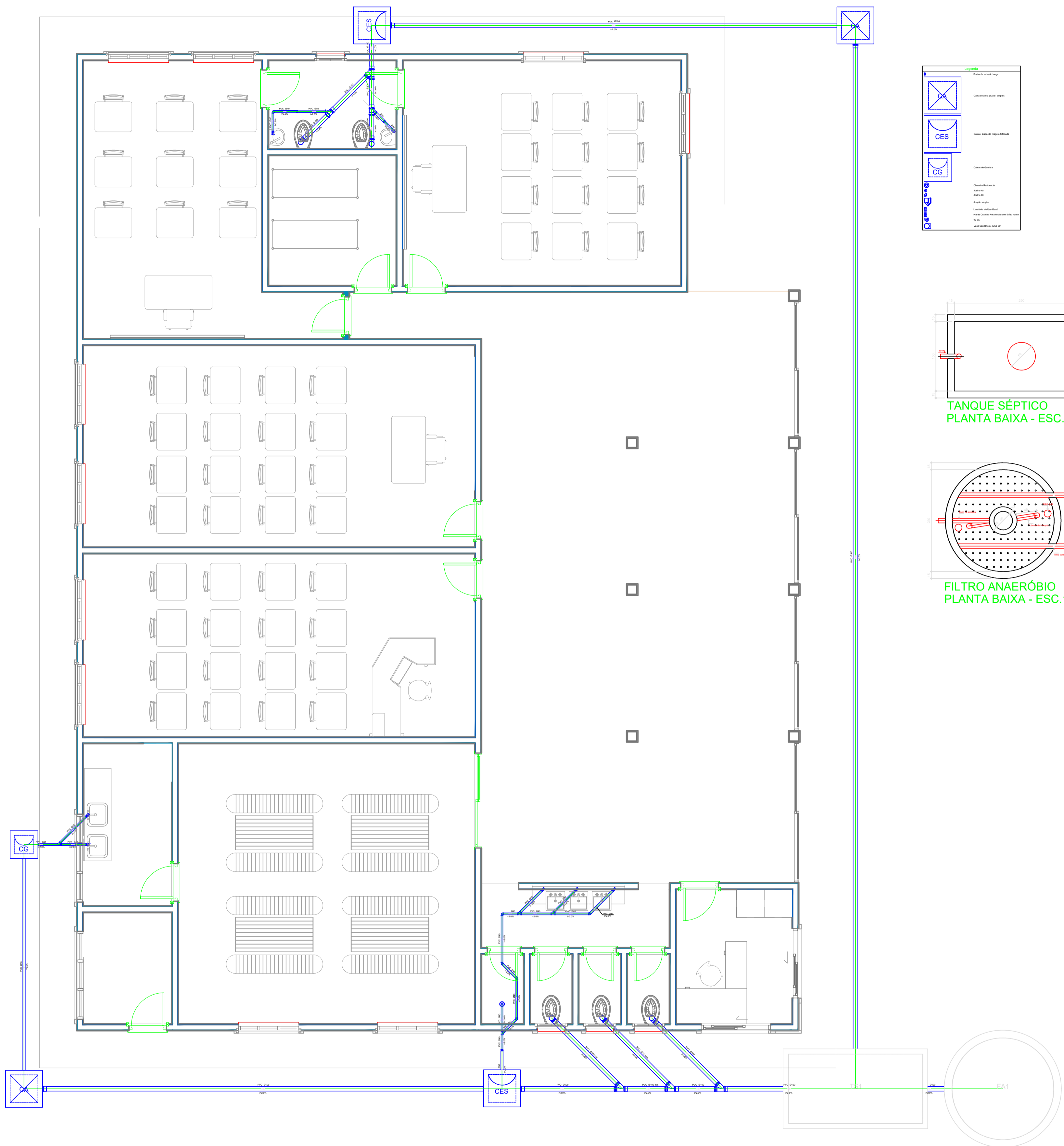
PLANTA BAIXA escala 1:50
