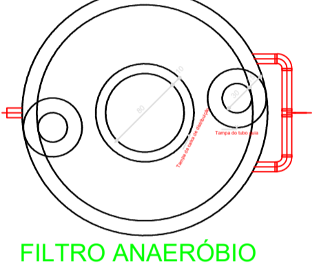
FILTRO ANAER BIO PLANTA BAIXA - ESC. 1:25
