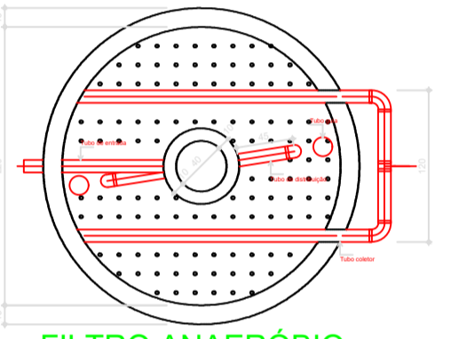
FILTRO ANAER BIO PLANTA BAIXA - ESC. 1:25
