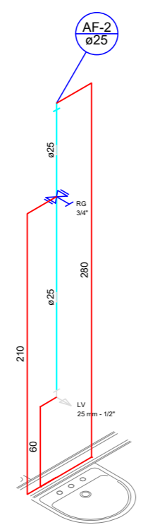
DETALHE AF-2 SEM ESCALA
