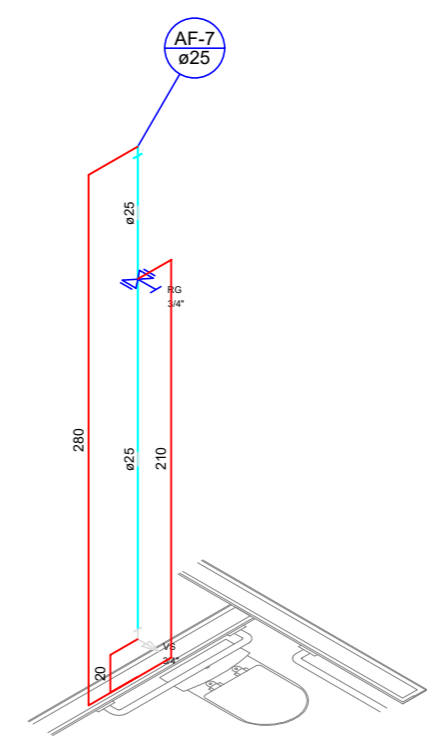
DETALHE AF-7 SEM ESCALA
