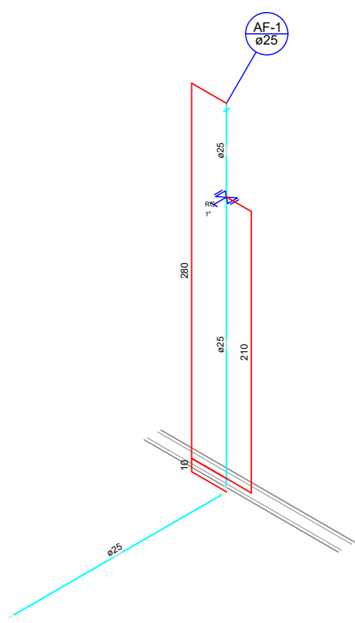
DETALHE AF-1 SEM ESCALA
