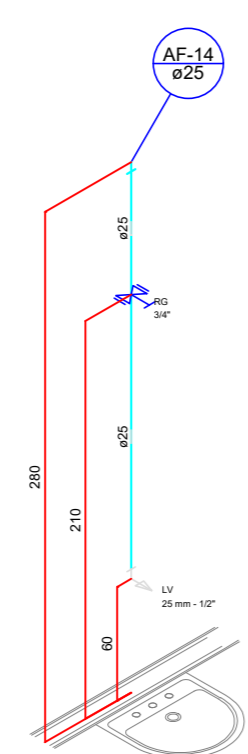
DETALHE AF-14 SEM ESCALA
