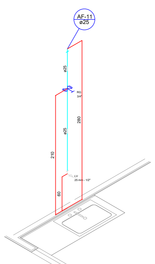
DETALHE AF-11 SEM ESCALA
