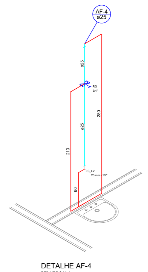
DETALHE AF-4 SEM ESCALA
