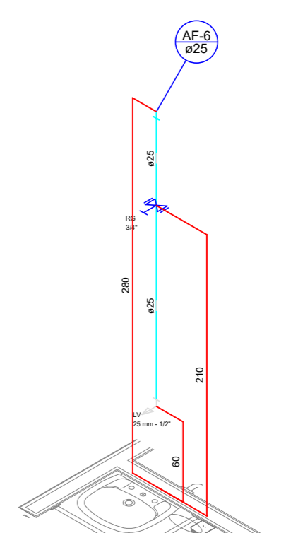
DETALHE AF-6 SEM ESCALA
