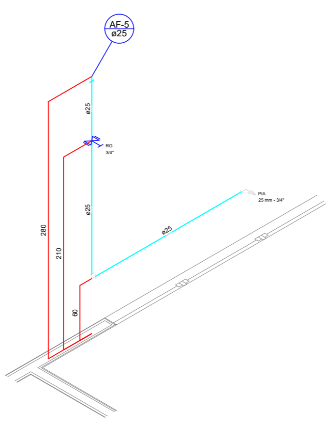
DETALHE AF-5 SEM ESCALA
