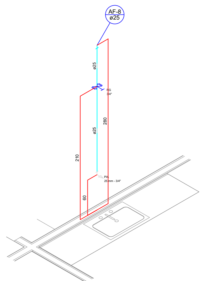
DETALHE AF-8 SEM ESCALA
