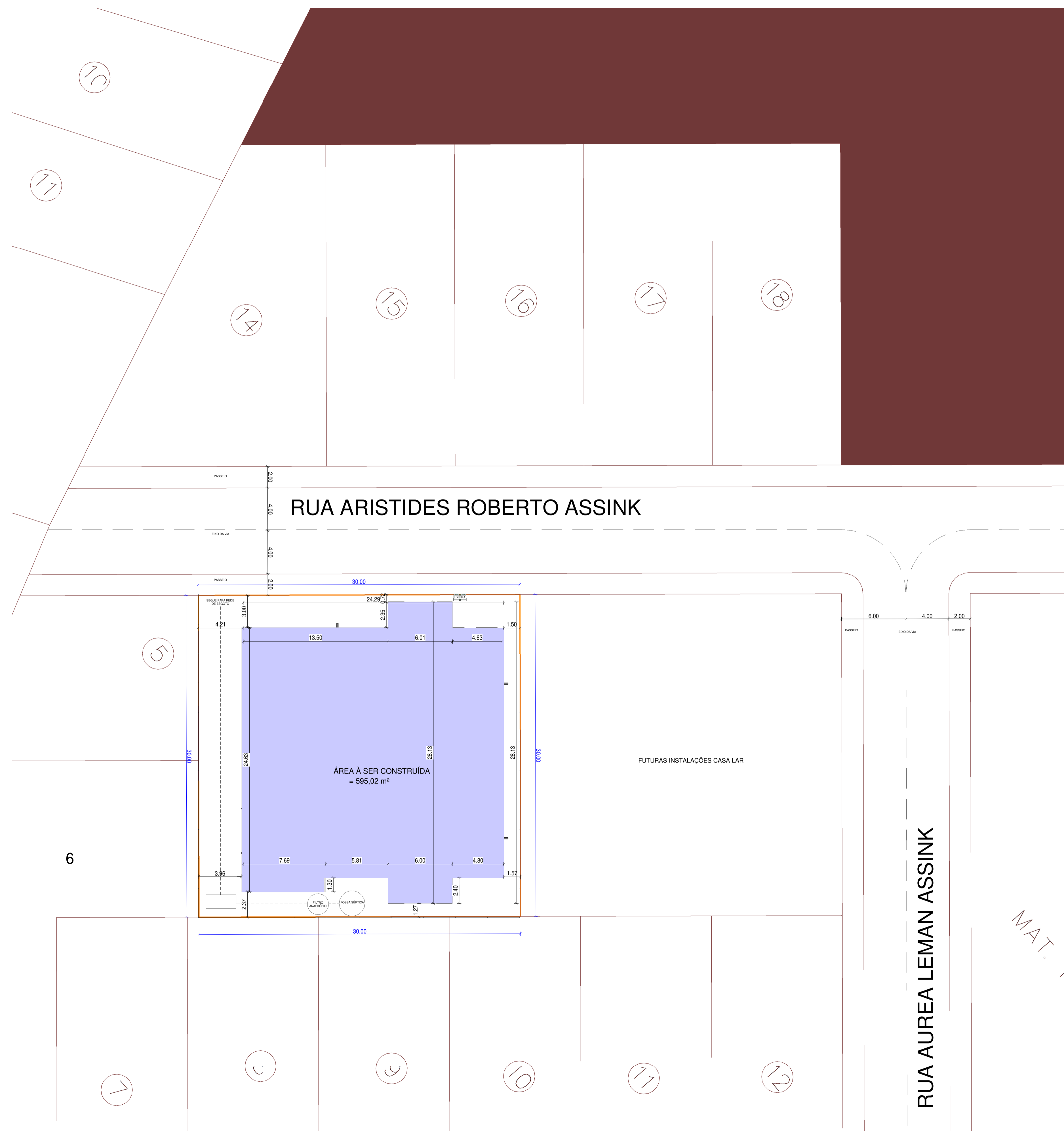
1 PLANTA DE SITUAÇÃO ESCALA 1:200
