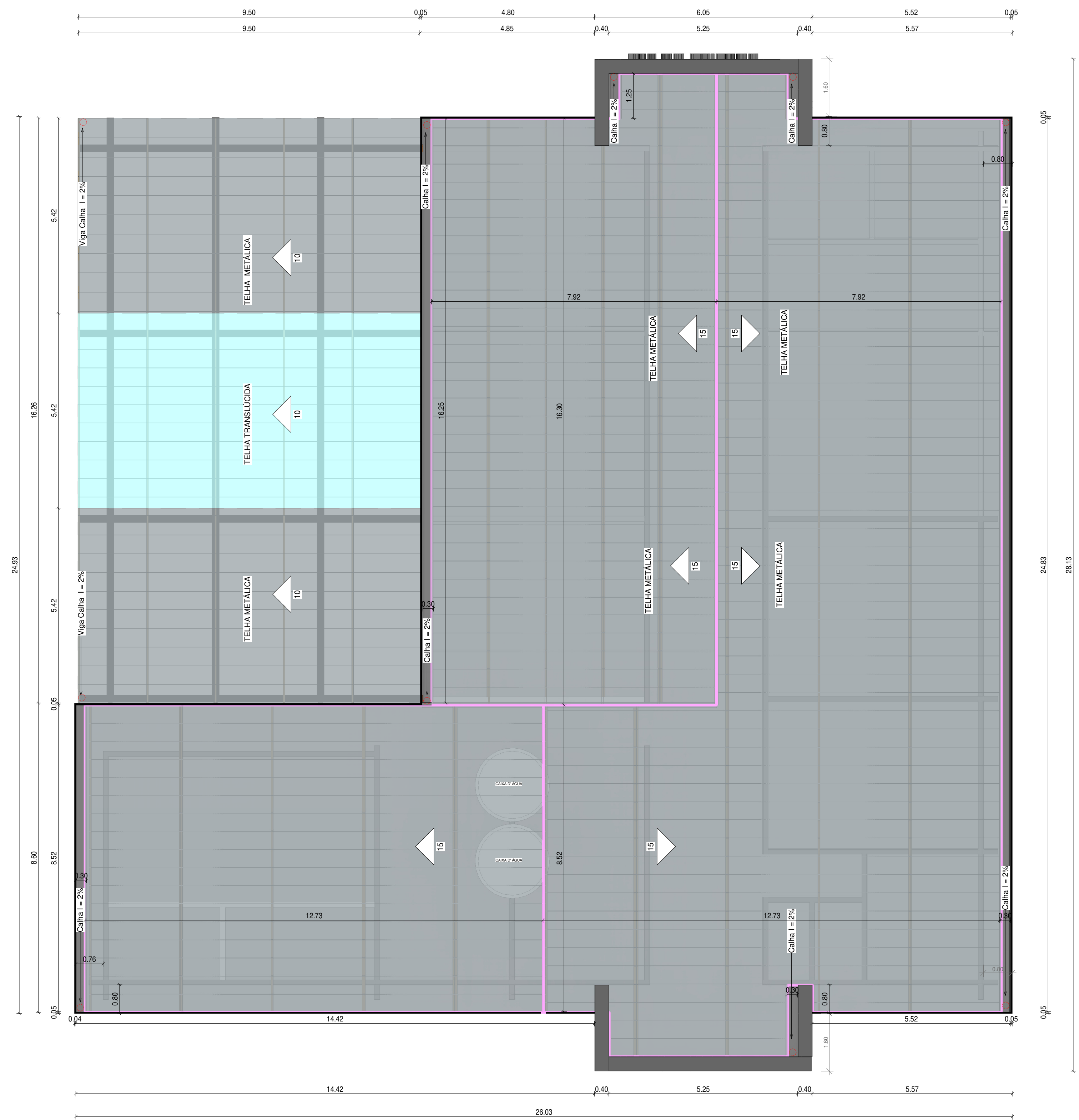
1 PLANTA DE COBERTURA ESCALA 1:75
