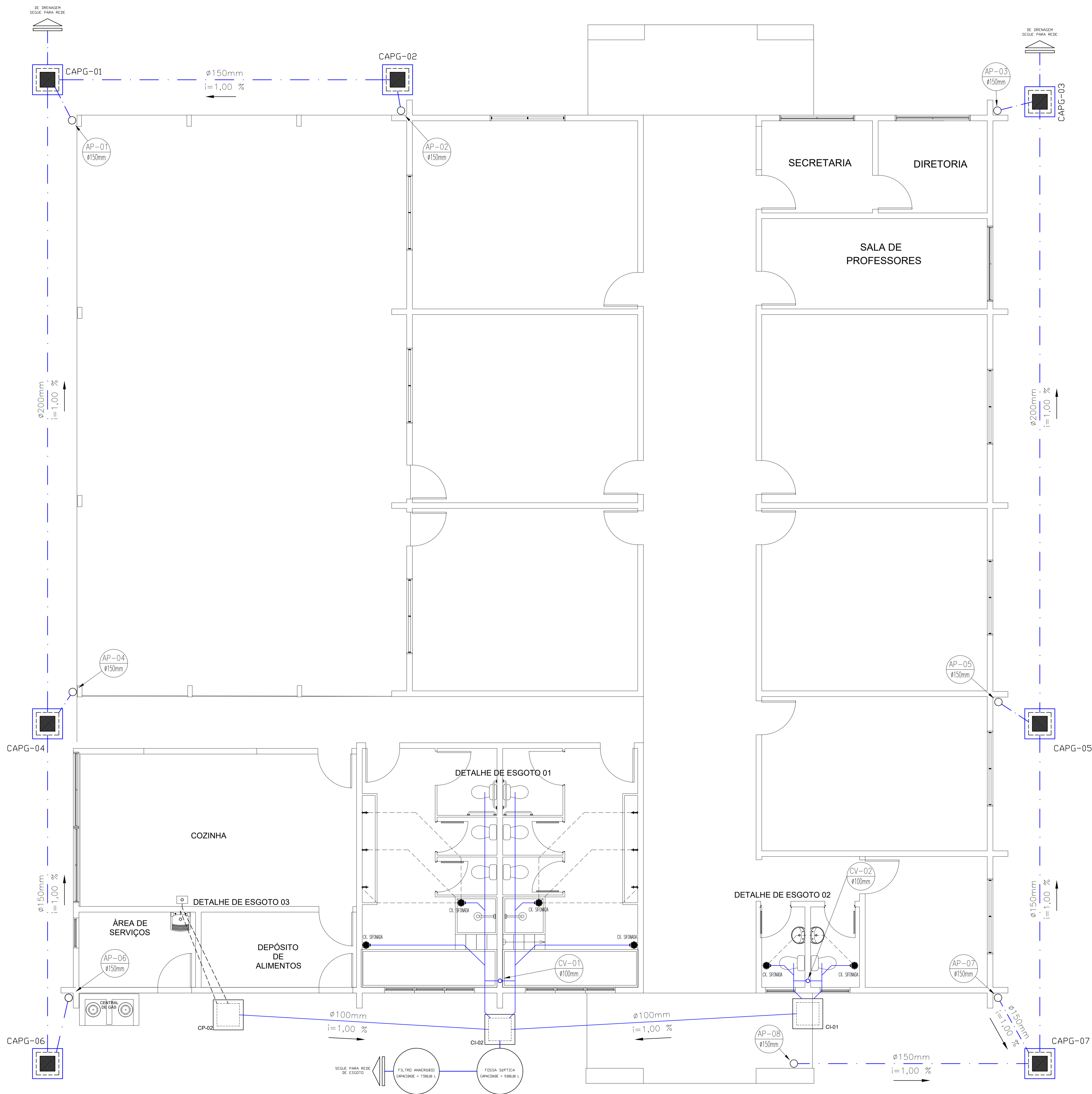
PLANTA BAIXA - CENTRO DE EDUCAÇÃO INFANTIL - ESGOTO / DRENAGEM ESC. 1/50
