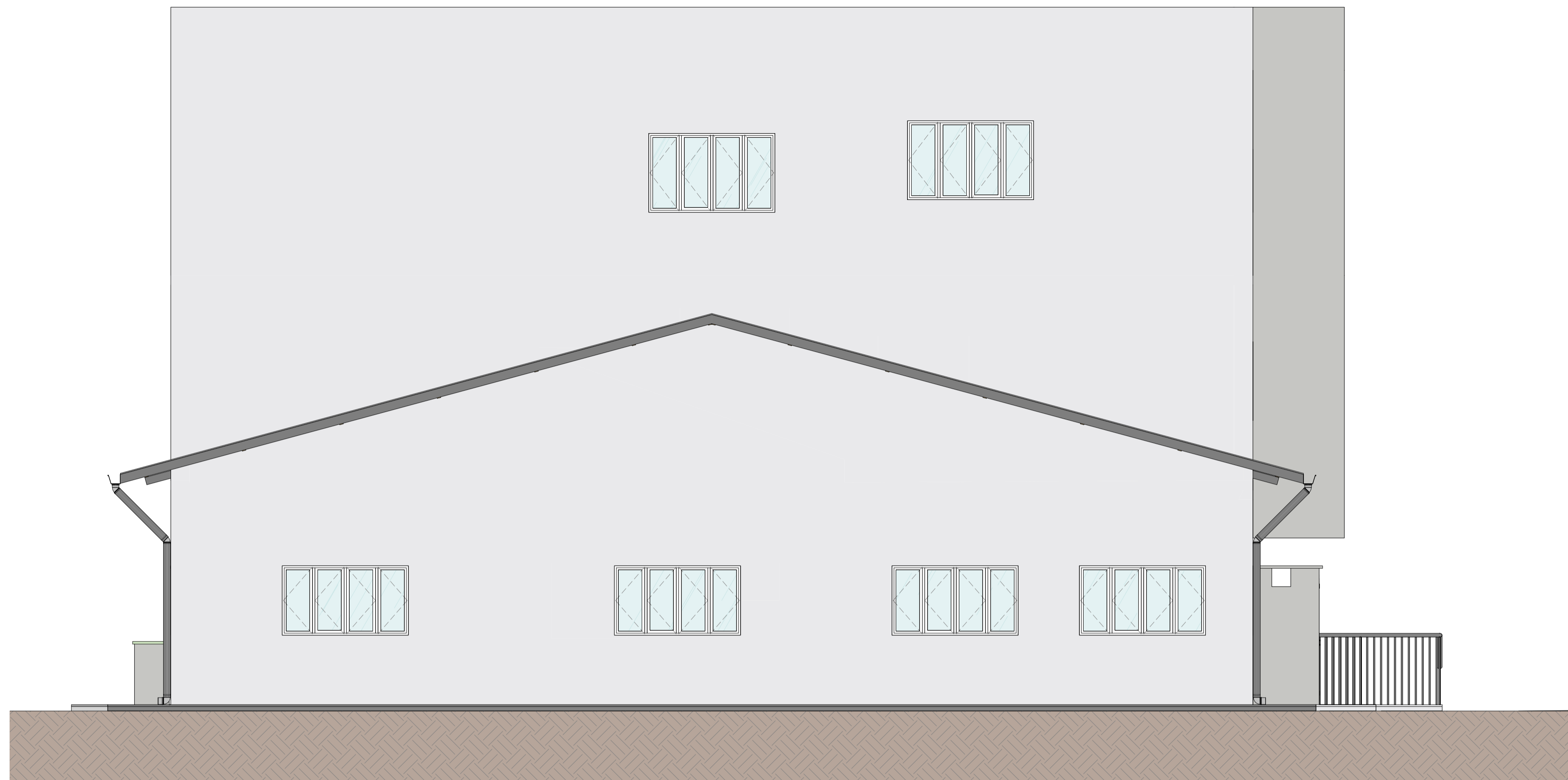
1 FACHADA LESTE 1 : 50
