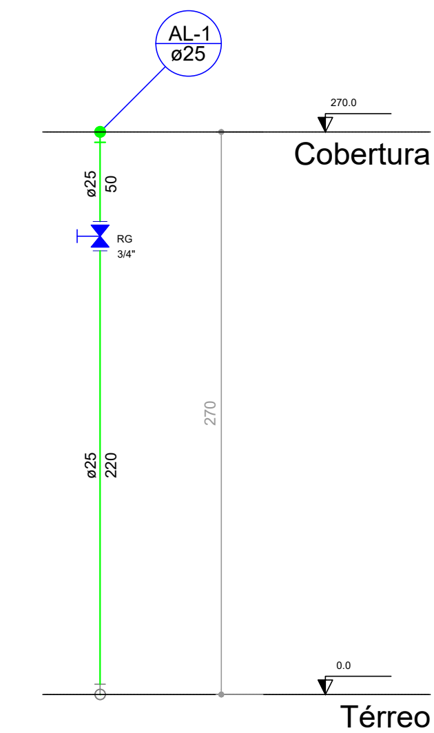
Corte Alimentação escala 1:25
