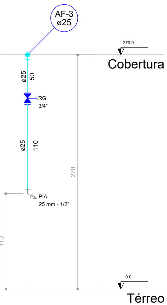
Corte Cozinha escala 1:25
