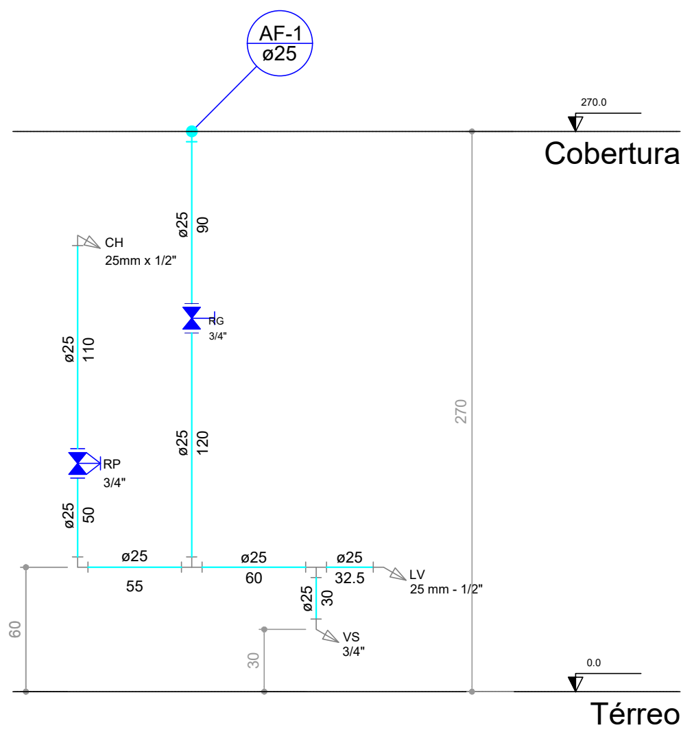
Corte Banheiro escala 1:25
