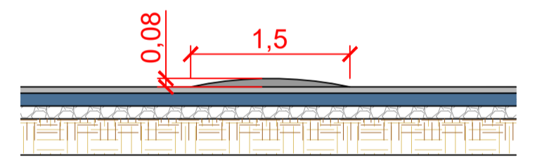
Detalhe Lombada
