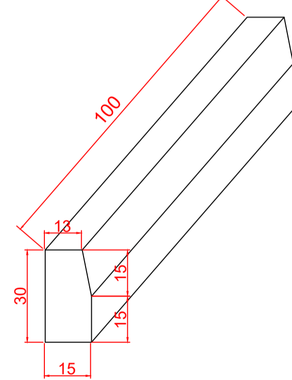
detalhe Meio-fio em concreto FCK= 25MPA
